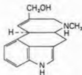
ELYMOCLAVINE
